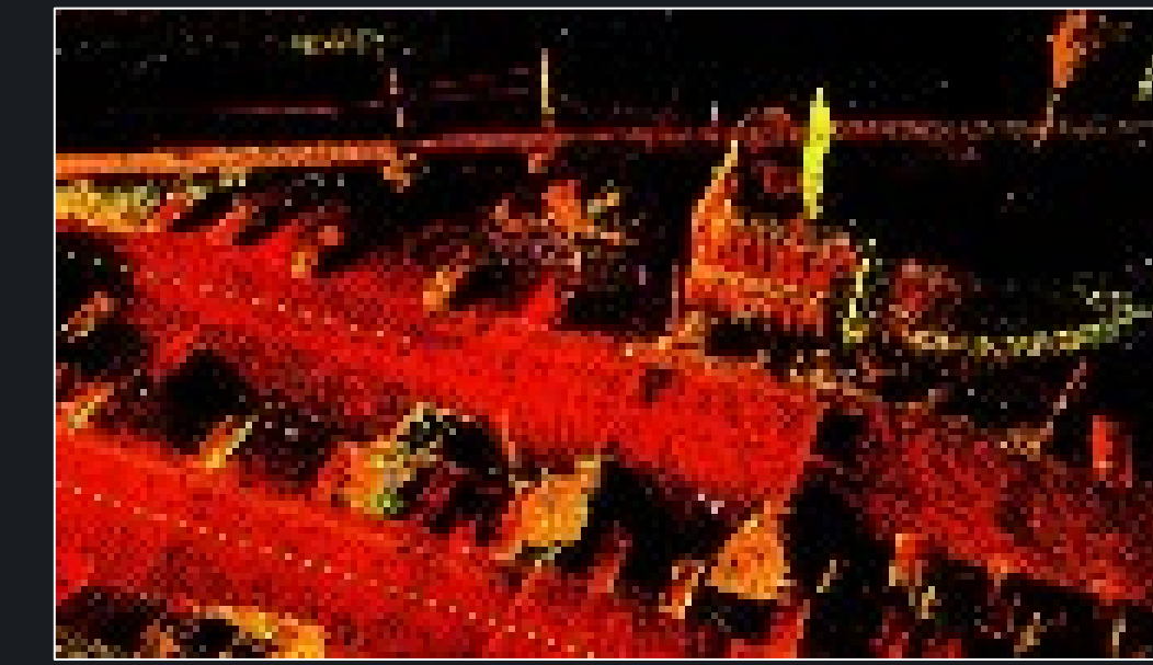
点云地图
